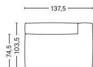
Left backrest Art. S9302 W137,5 x D74,5/103,5 x H37/67 cm
