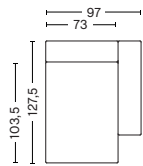
Right armrest* Art. 8161 W73/97 x D103,5/127,5 x H40/67 cm Armrest D24 cm
