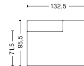
Left backrest Art. 9302 W132,5 x D71,5/95,5 x H40/67 cm
