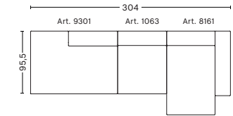
W304 x D95,5/127,5 x H40/67 cm
